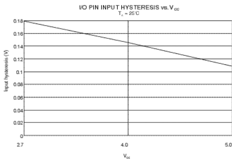
图 52 I/O 引脚输入容限与电压的关系
