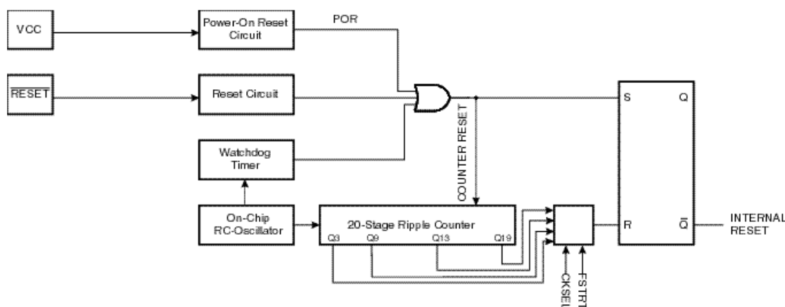
图 16 ATtiny10/11 的复位逻辑
