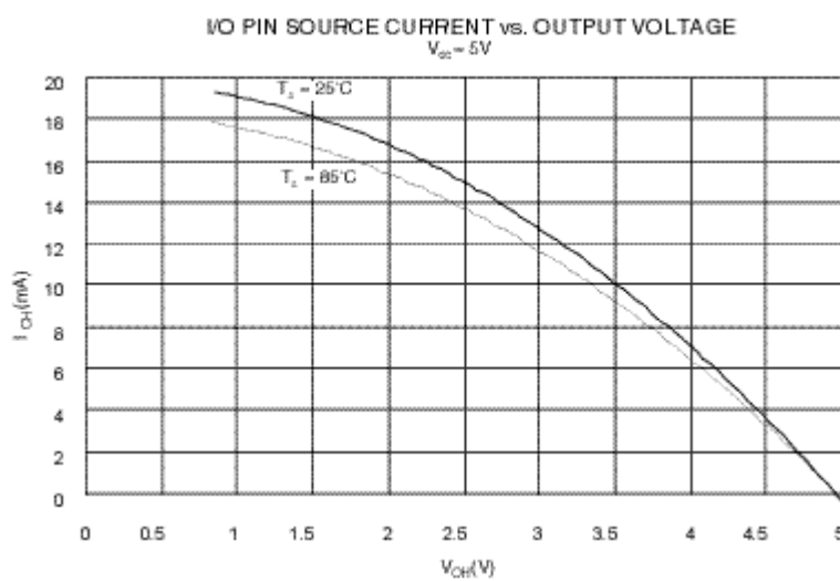
图 54 I/O 引脚输出电流与输出电压的关系
