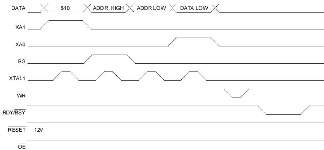
图 32 编程波形二
