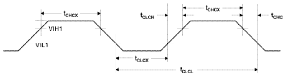
图 37 外部时钟
