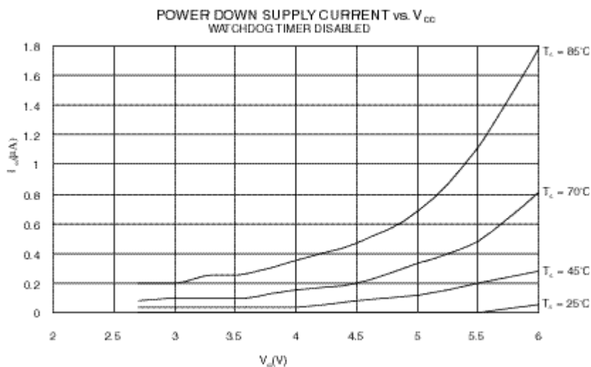
图 44 工作电流与电压的关系， 掉电模式， 看门狗禁止
