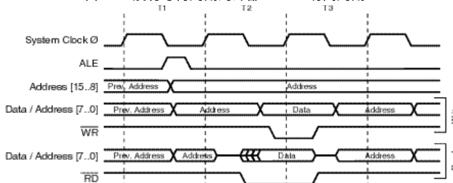
图 44 有等待周期的外部 SRAM 访问周期
