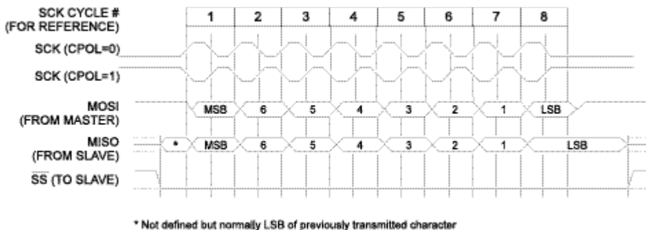
图 37 SPI 传输格式 (CPHA=1, DORD=0)
