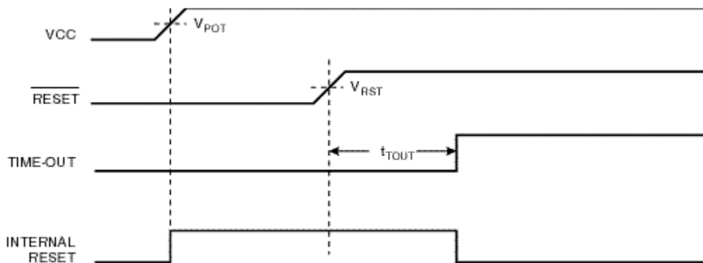
图 25 MCU 启动，/RESET 由外电路控制
