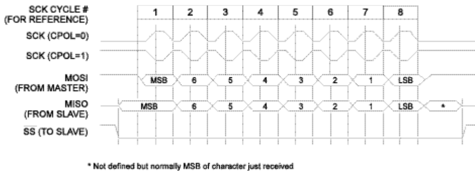
图 36 SPI 传输格式 (CPHA=0, DORD=0)
