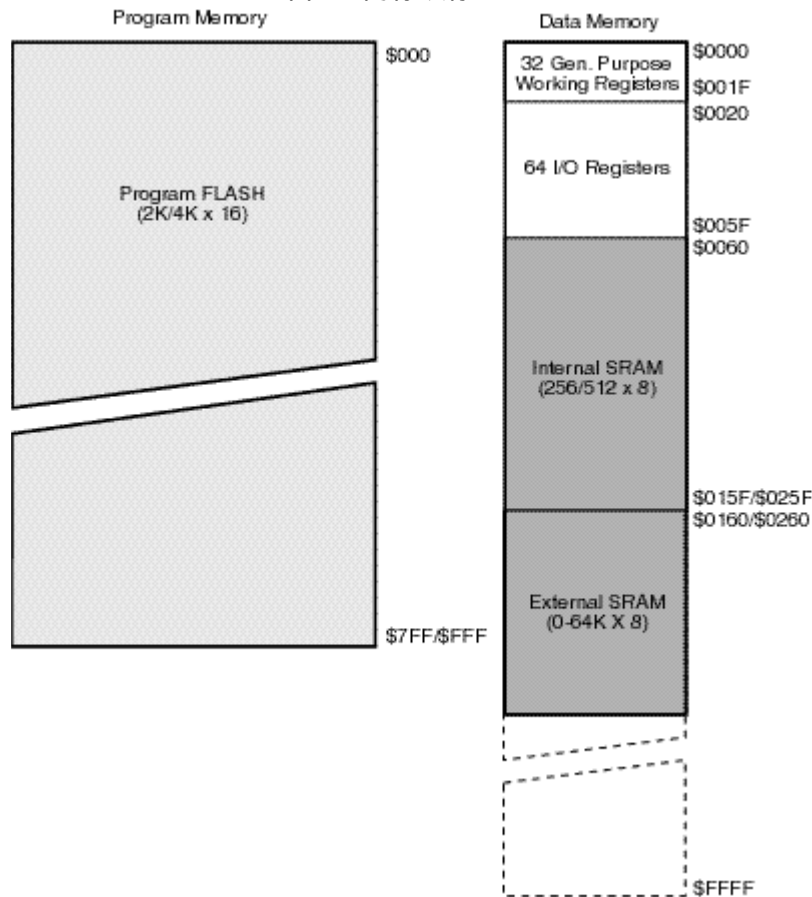
图 5 内存映像
