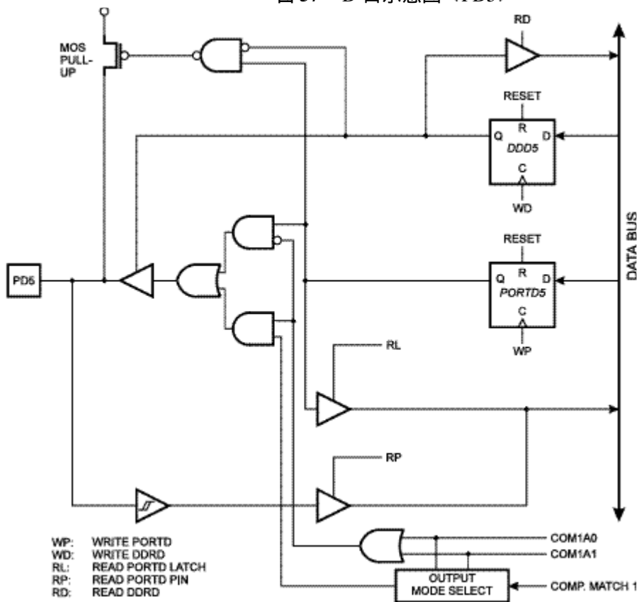
图 57 D 口示意图 (PD5)
