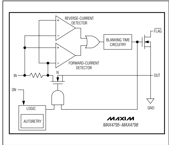
图1. 原理框图
