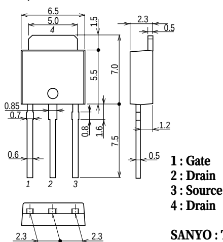
外形図 2083B
