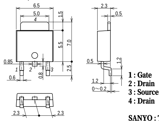
外形図 2092B
