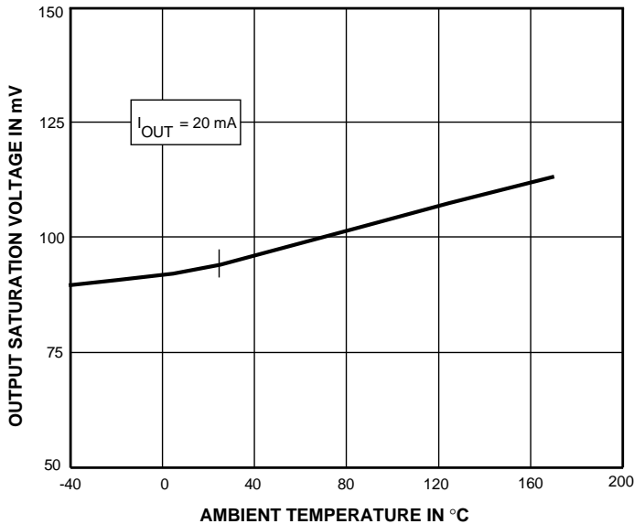
Dwg. GH-013-1
