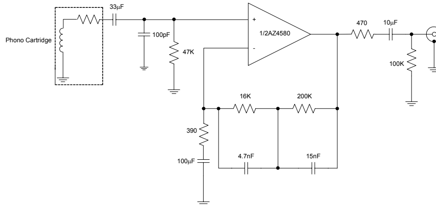
Figure11. RIAA Preamp
