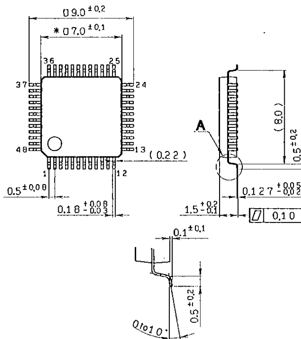
VQFP-48P-L01
