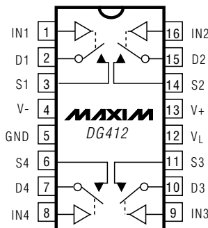
DIP/SO/TSSOP
