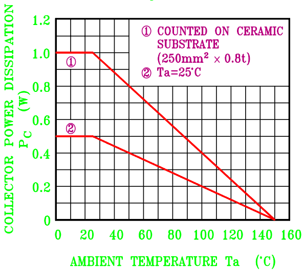
P_C - T_a
