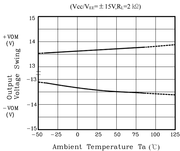
Fig. 7 V_{OM} - T_a
