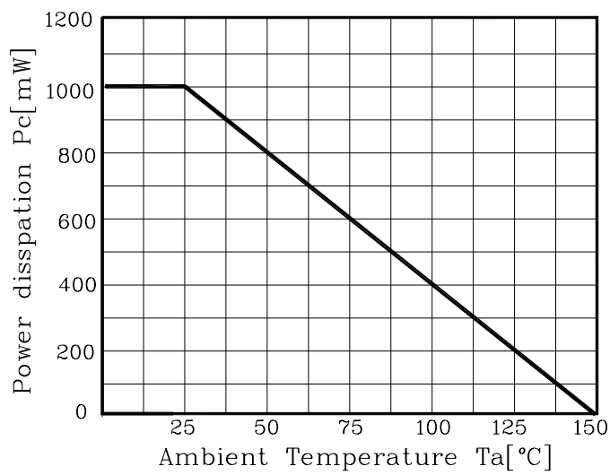
Fig. 3. P_d - T_a
