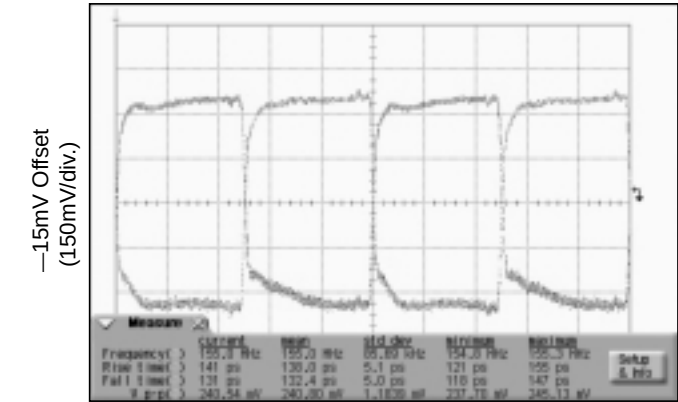
155MHz Output
