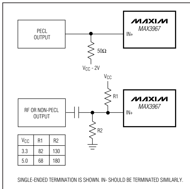
图 3. 输入端接
