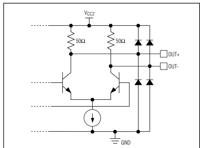
图 6. OUT+/OUT- 等效输出结构
