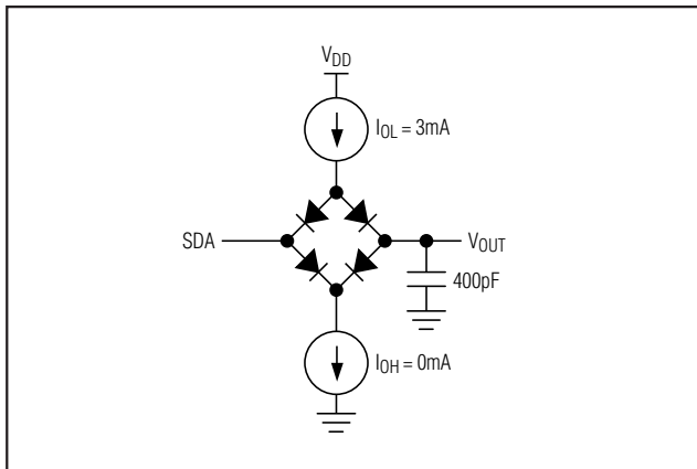
图 2. 负载电路
