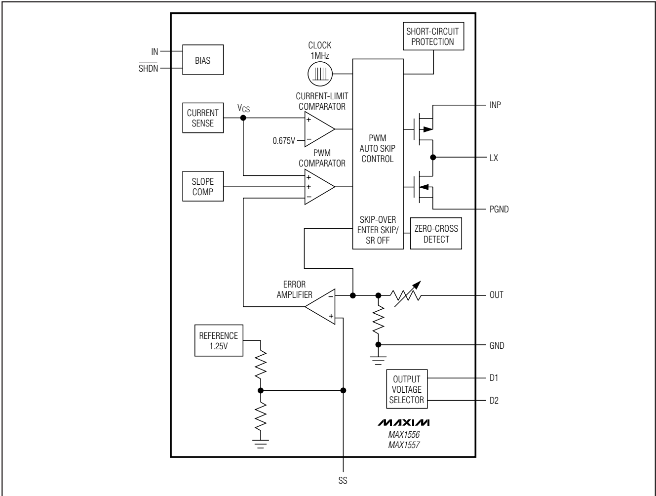
图1. 功能框图
